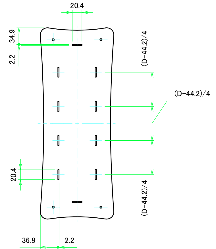
上カバー裏面 / Top cover Backside
