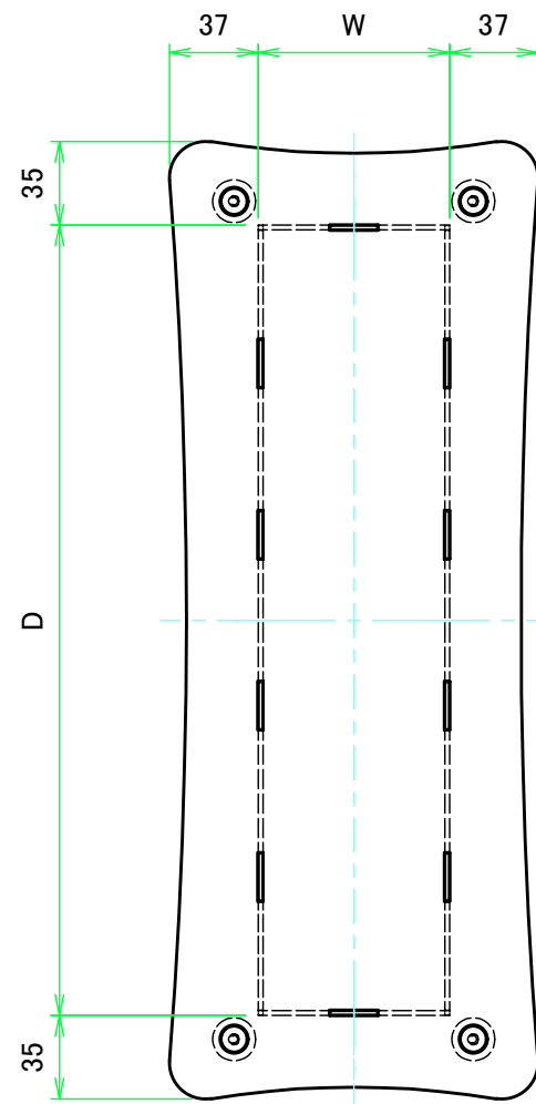
上カバー / Top cover
