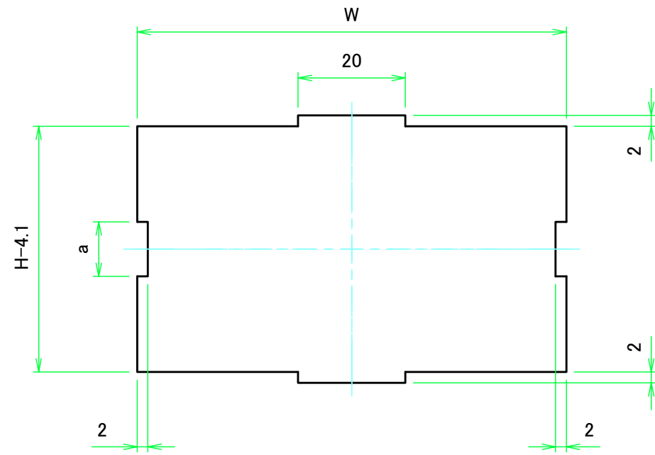
Wパネル1表面 / W panel 1 Frontside
